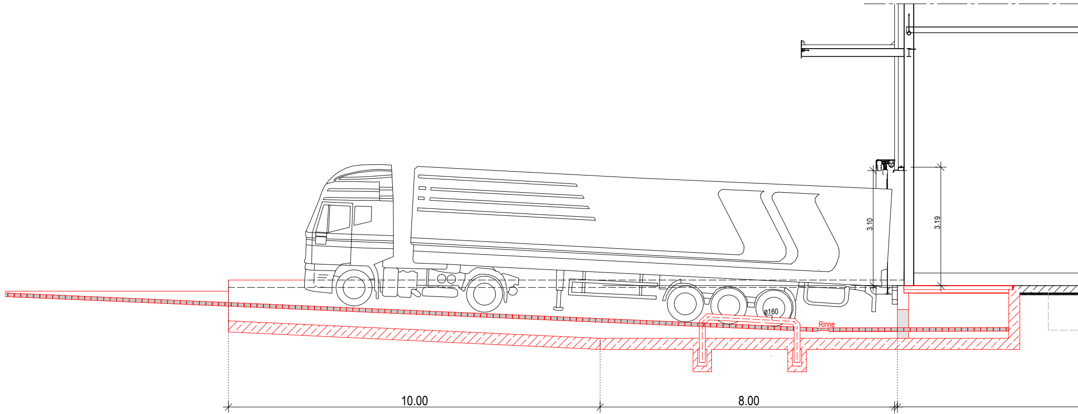
Schnitt G - G
