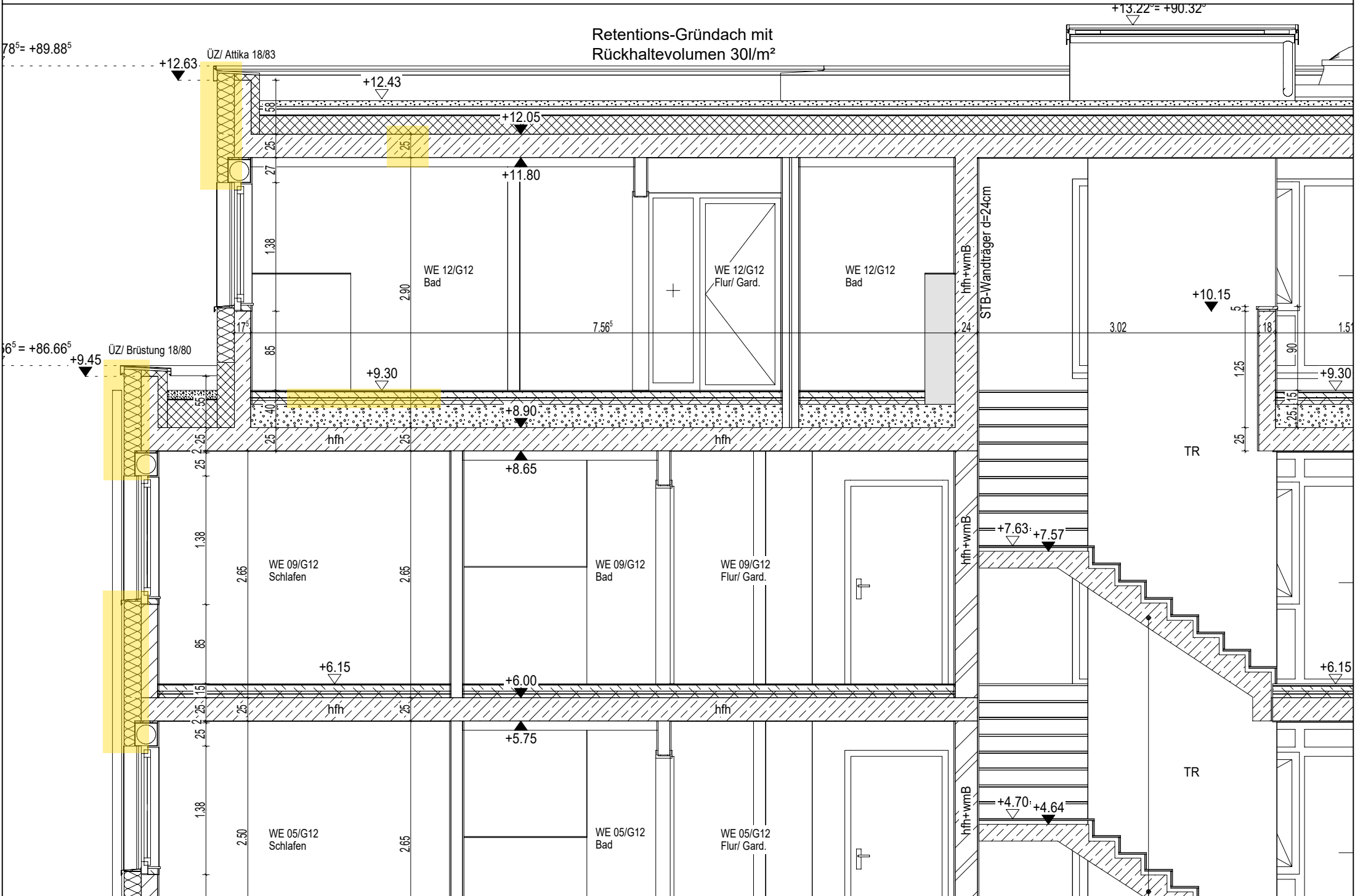
Schnitte/9300_Schnitte/ Ansichten/Gebäude 12/G12 AP-Schnitte M 1 : 50
