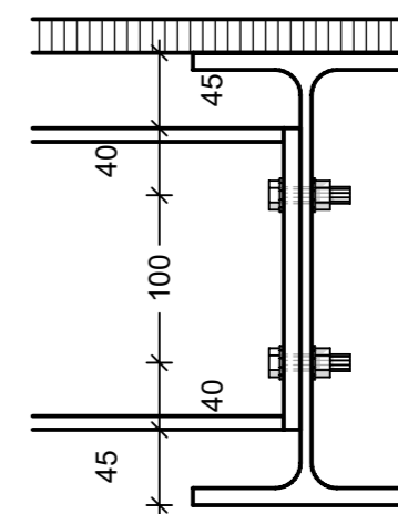
Détail assemblage IPE180 - IPE270 ech : 1:5 cotations en mm
